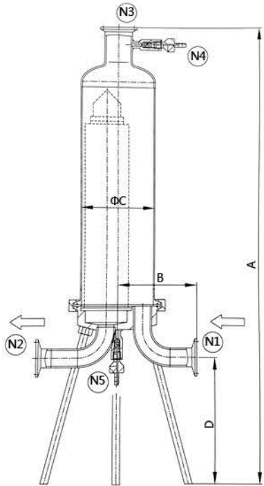
单芯卫生级液体过滤器 ( 222 型、226 型 ) Single fluid sanitary filter housing (222tpe、226type)
