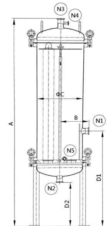
精密液体过滤器（滤芯数量 \leq 12 芯） 滤芯型号为 30" 滤芯（左图示） Precision Liquid Filter (cartridge quantity \leq 12 pcs) Cartridge model 30" (left picture)
