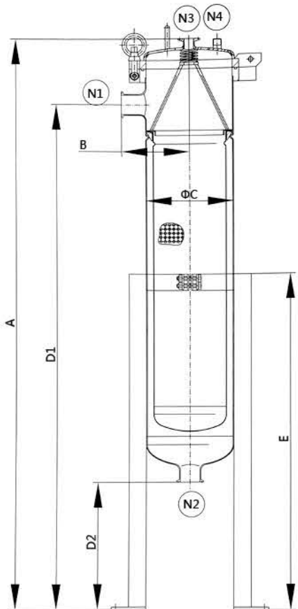
侧入式袋式过滤器 Side entry bag filter
